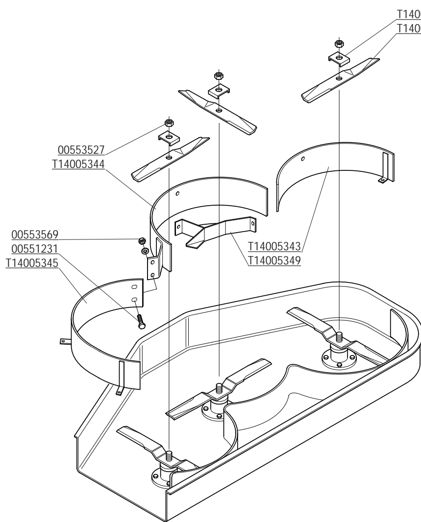
SCARICO LATERALE
